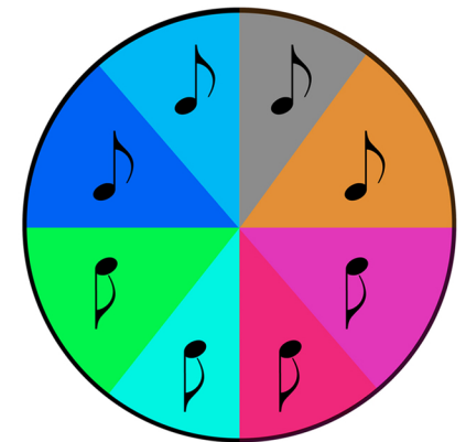
ACHTELKUCHEN = ACHTELNOTE
